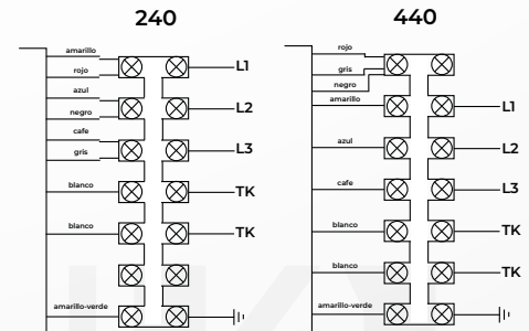
DIAGRAMA DE CABLEADO
